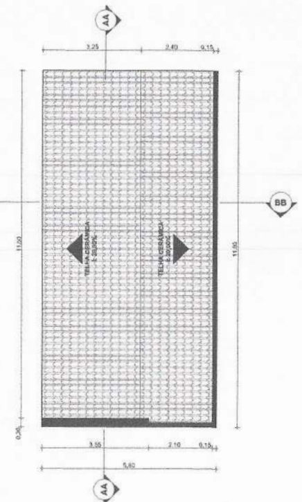
4 COBERTA Escala: 1:120
